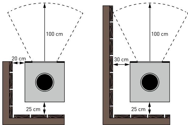
Draufsicht Brennkammer
