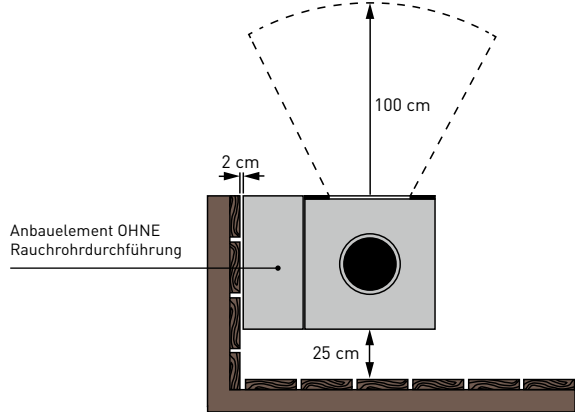
Draufsicht Brennkammer
