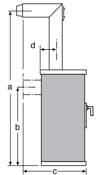
Maß a und c: mit Original-Winkelrohr dimension a and c: with original angle pipe misura a e c: con tubo ad angolo originale câtes a et c: avec conduit caudé d'origine
